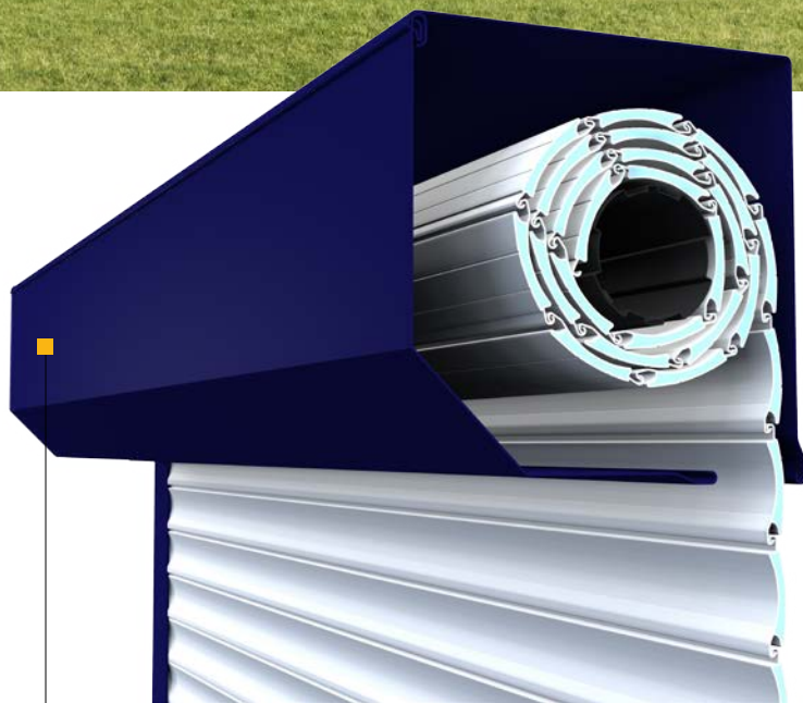
Coffre extérieur CLASSIQUE avec pan coupé
