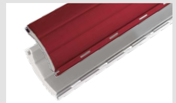
LAME ALUMINIUM Eco-Energie 43 mm Lame à 2 faces différentes avec une face aluminisée tournée vers l'intérieur qui limite les pertes d'énergie. Éligible au CRÉDIT D'IMPÔT selon règle fiscale en vigueur.
